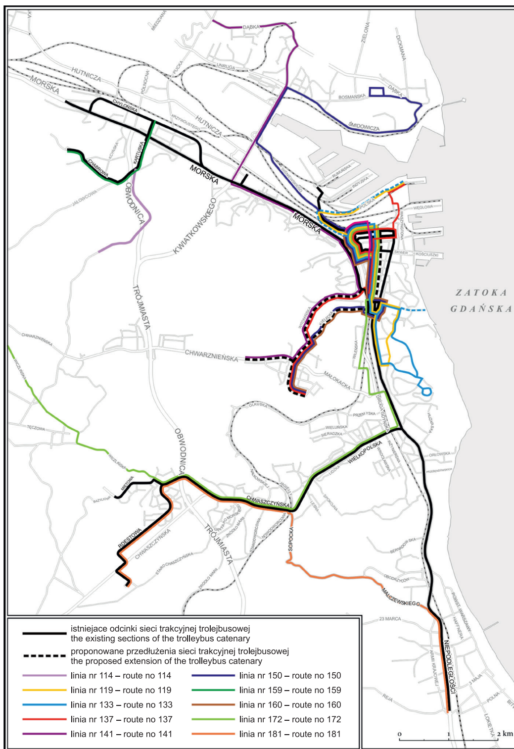
Rys. 1. Schemat linii autobusowych wyznaczonych jako potencjalne do obsługi trolejbusami z bateriami Fig. 1. Diagram of the bus routes designed as potential to use trolleybuses with batteries
