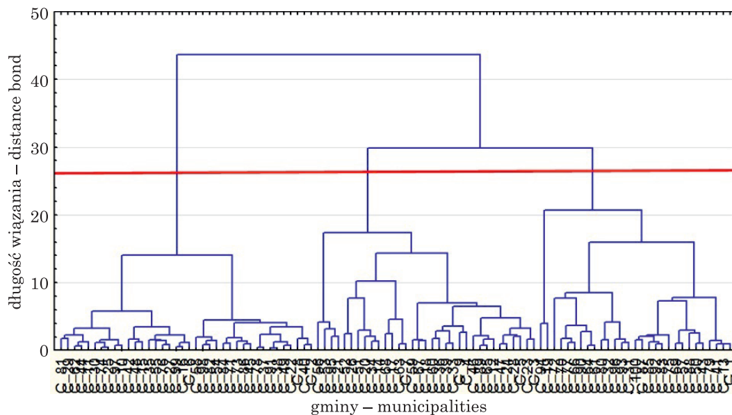
Rys. 1. Dendrogram drzewa powstały z użyciem metody Warda
